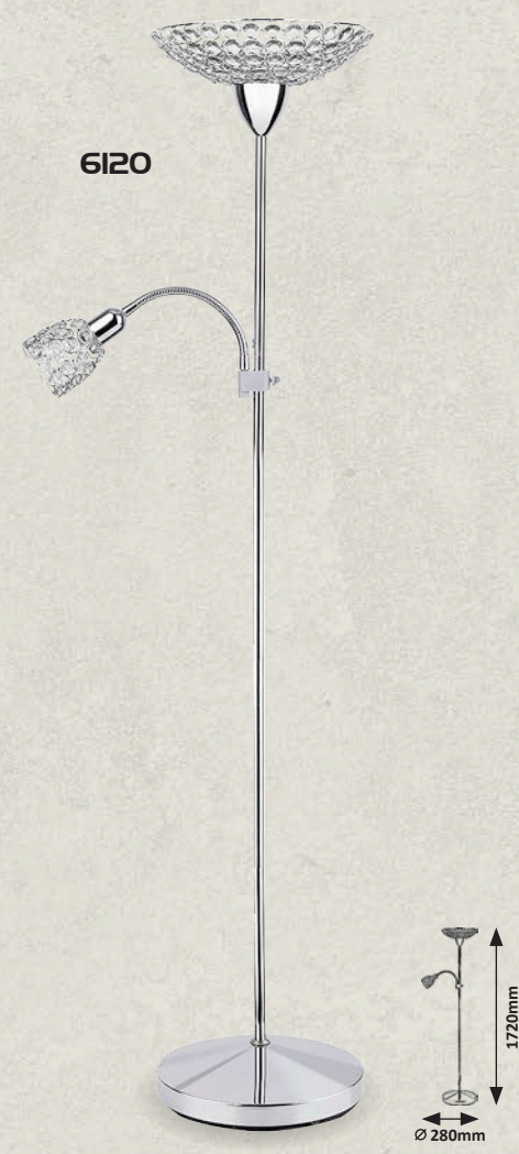
6120 MGC ☒ E-27 / G45 / 1x max. 60W + E-14 / 1x max. 40W IP20 • • chrome/crystal
