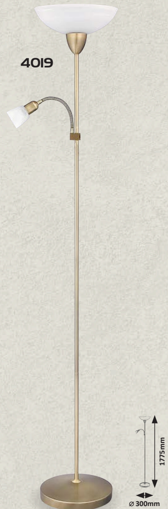
4019 MG ☒ E-27 / G45 / 1x max. 60W + E-14 / 1x max. 40W IP20 • • 9585 • 9584 bronze/alabaster
